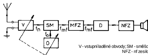
Obr. 144. Blokové schéma superhetu
