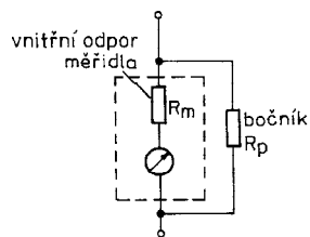
Obr. 211. Úprava rozsahu ampérmetru bočníkem
