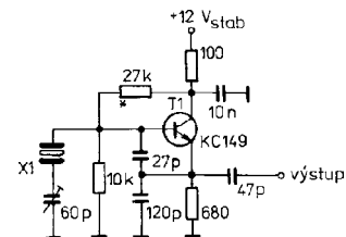
Obr. 93. Příklad zapojení krystalového oscilátoru
