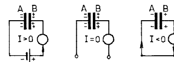
Obr. 16. Nabíjení a vybíjení kondenzátoru
