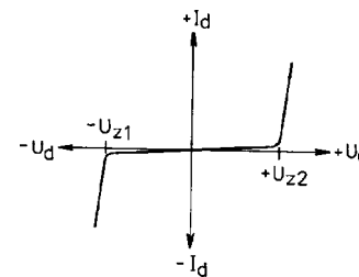
Obr. 113. Příklad omezovače vf napětí využívajícího charakteristiky dvou Zenerových diod s opačnou polaritou v sériovém zapojení
