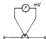
Obr. 212. Termoelektrický článek pro měření v_f proudu
