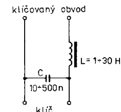
Obr. 160. Příklad jednoduchého klíčovacího filtru
