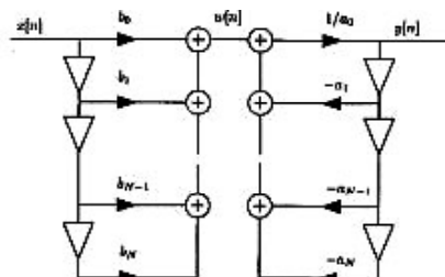
Obr. 154. Přímá realizační struktura
