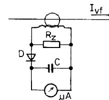
Obr. 213. Transformátor k měření v_f proudu na KV
