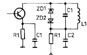
Obr. 113. Příklad omezovače vf napětí využívajícího charakteristiky dvou Zenerových diod s opačnou polaritou v sériovém zapojení
