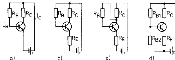
Obr. 68. Nastavení a stabilizace pracovního bodu:
