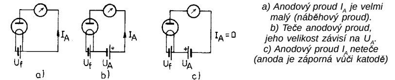
Obr. 54. Princip usměrňovacího efektu vakuové diody:
