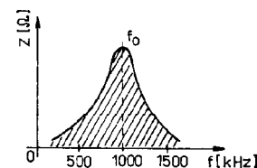
Obr. 117. Kmitočtová závislost impedance paralelního LC obvodu
