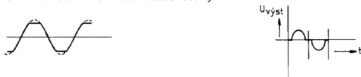
Obr. 80. Jiný příklad nelineárního zkreslení dvojčinného zesilovače třídy B při malé amplitudě
