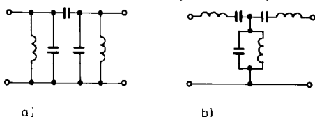
Obr. 135. Jednoduché varianty zapojení pásmových propustí
