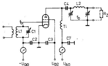
Obr. 172. Koncový vř zesilovač s elektronkou v zapojení se společnou katodou pro KV pásma
