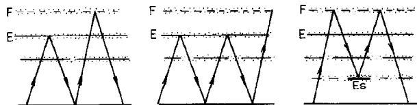
Obr. 238. Využití kombinace odrazů od různých vrstev ionosféry
