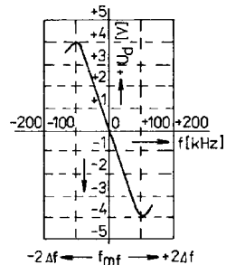
Obr. 107. Příklad demodulační charakteristiky demodulátoru FM jako závislosti výstupního nf signálu na kmitočtovém zdvihu
