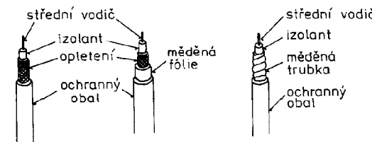
Obr. 179. Různá provedení souosých kabelů
