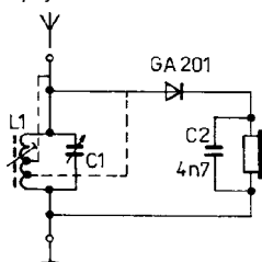
Obr. 142. Zapojení jednoduchého diodového přijímače bez zesílení
