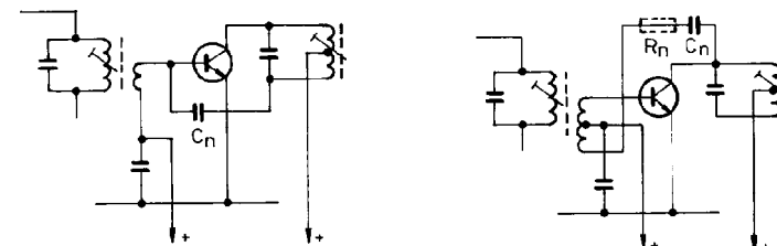
Obr. 90. Příklad zapojení neutralizace
