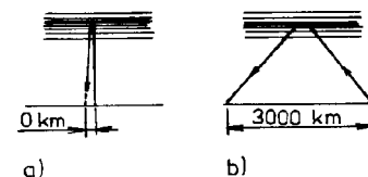
Obr. 236. Kritický kmitočet a) a maximální použitelný kmitočet b) o
