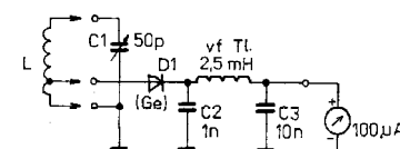
Obr. 222. Absorpční vlnoměr
