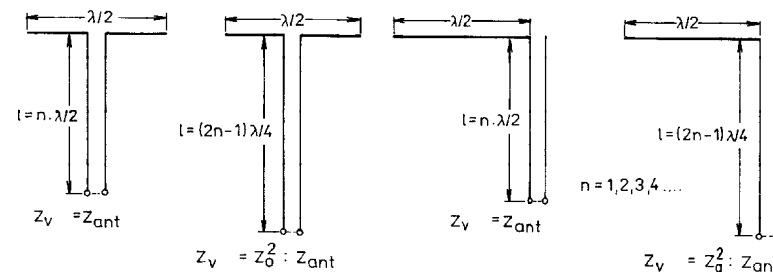
Obr. 183. Různé varianty napájení půlvlnného dipólu
