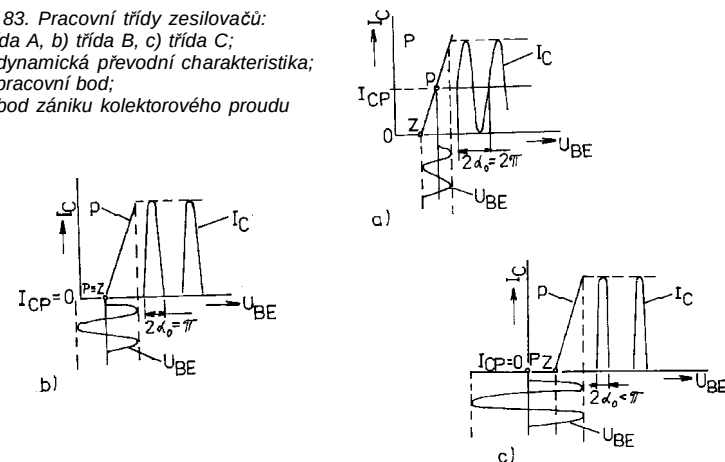
Obr. 83. Pracovní třídy zesilovačů:
