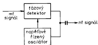
Obr. 150. Princip demodulátoru s fázovým závěsem
