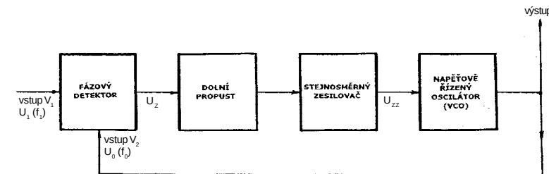
Obr. 148a. Základní blokové schéma fázového závěsu (PLL)
