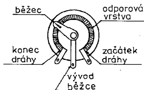
Obr. 12. Proměnný rezistor - potenciometr
