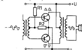
Obr. 85. Dvojčinné zapojení zesilovače třídy B
