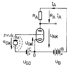
Obr. 58. Příklad základního zapojení zesilovacího stupně s triodou. Zesílený signál vzniká na pracovním anodovém rezistoru R_A
