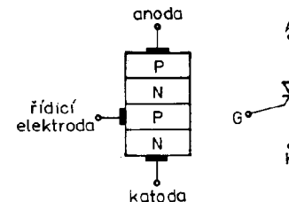
Obr. 70. Struktura tyristoru a jeho schematická značka
