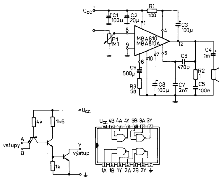
Obr. 75. Elektrické zapojení a patice integrovaného obvodu MH7400
