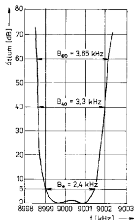
Obr. 149. Příklad křivky propustnosti solidního filtru soustředěné selektivity
