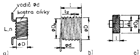
Obr. 23. Příklady skutečného provedení cívky:
