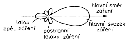
Obr. 187. Příklad horizontálního vyzařovacího diagramu směrové antény
