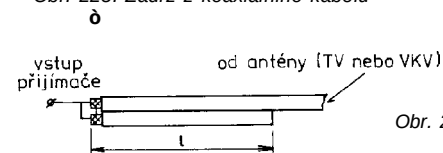
Obr. 225. Zádrž z koaxiálního kabelu
