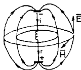
Obr. 41. Princip vzniku elektromagnetického pole
