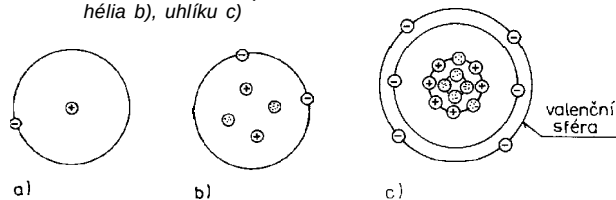
Obr. 1. Atom vodíku a), hélia b), uhlíku c)
