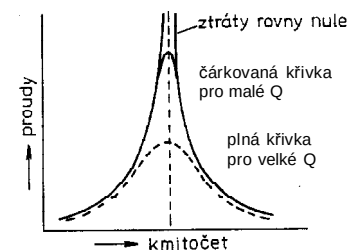
Obr. 35. Průběh proudu sériového LC obvodu v závislosti na kmitočtu a činiteli jakosti
