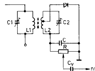
Obr. 99. Sériový detektor pro demulaci amplitudově modulovaných signálů
