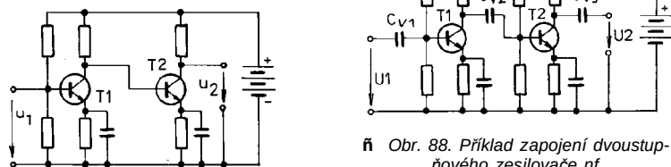
Obr. 87. Příklad zapojení dvoustupňového zesilovače se stejnosměrnou vazbou
