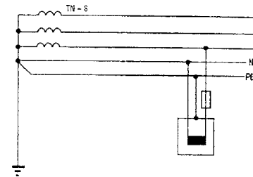
Obr. 247. Elektrorozvodná soustava TN-S
