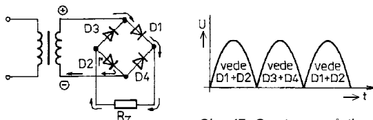
Obr. 47. Graetzovo můstkové zapojení dvoucestného usměrňovače a průběh výstupního napětí
