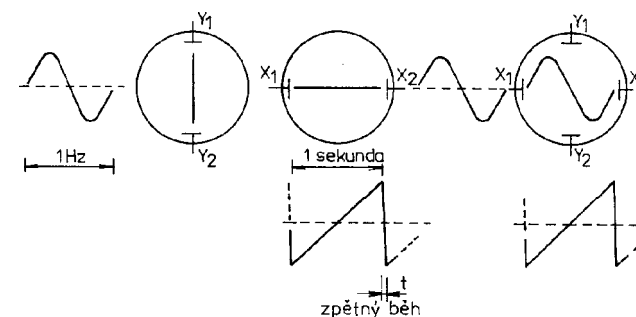
Obr. 224 . Princip vychylování paprsku na osciloskopu
