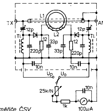
Obr. 221. Příklad zapojení měřiče ČSV pro krátké vlny \delta
