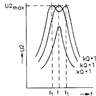
Obr. 125. Různý tvar přenosové křivky dvou vzájemně vázaných LC obvodů při různých hodnotách k \cdot Q_0
