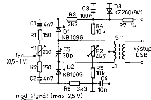
Obr. 164. Zapojení modulátoru s dvěma varikapky
