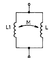
Obr. 25. Paralelně zapojená dvojice indukčně vázaných cívek
