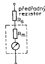
Obr. 214. Změna rozsahu voltmetru o předřadným rezistorem
