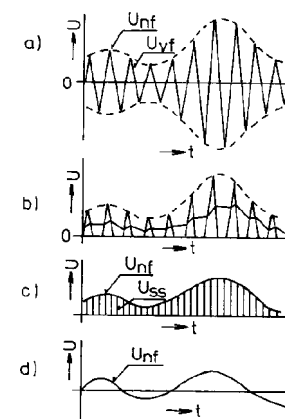
Obr. 100. Princip detekce signálů AM
