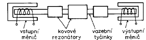
Obr. 128. Principiální sestava elektromechanického filtru
