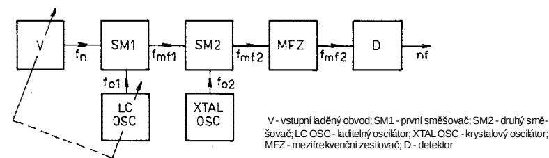
Obr. 145. Blokové schéma superhetu s dvojím směšováním
