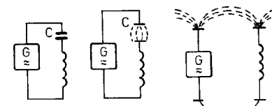
Obr. 40. Vznik otevřeného kmitavého obvodu s anténou
