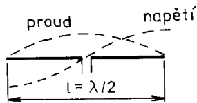
Obr. 194. Rozložení proudu a napětí na půlvlnném dipólu
