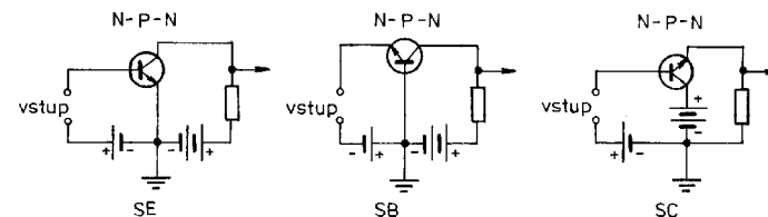
Obr. 66. Tři základní zapojení bipolárního tranzistoru
