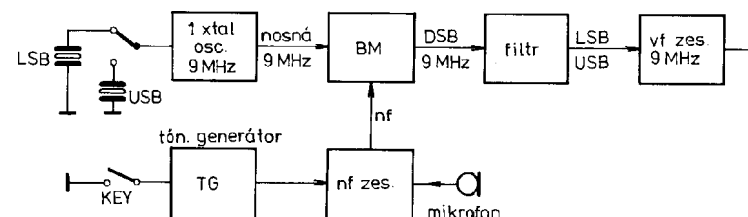
Obr. 163 Blokové schéma základního budiče SSB signálů
