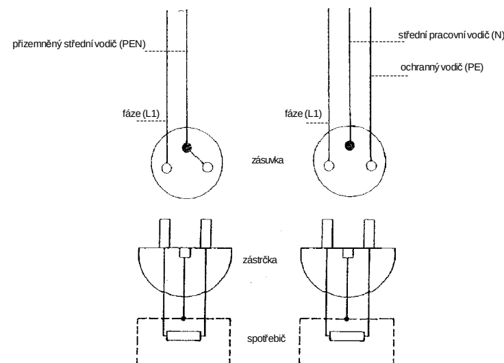
Obr. 249. Zásuvka a zástrčka jednofázového rozvodu TN-C a nového rozvodu TN-S
