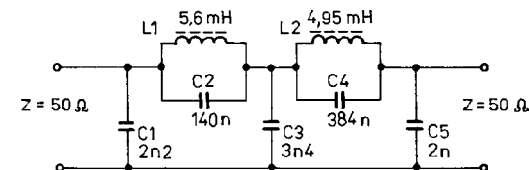
Obr. 167. Zapojení dolní propusti se zlomovým kmitočtem 1,8 kHz
