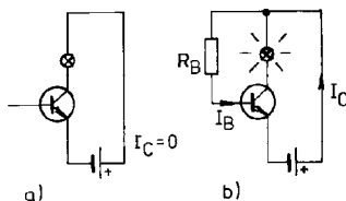
Obr. 65. Tranzistor NPN jako zesilovač proudu
