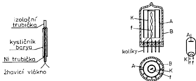
Obr. 52. Nepřímo žhavená katoda
