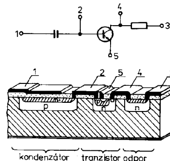
Obr. 72. Část polovodičového integrovaného obvodu, který obsahuje kondenzátor, tranzistor a rezistor
