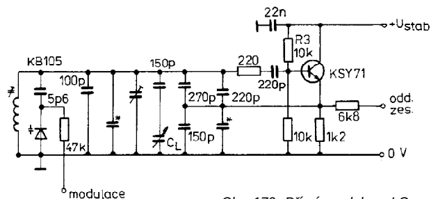
Obr. 170. Přímá modulace LC oscilátoru varikapem
