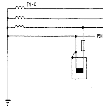
Obr. 246. Elektrorozvodná soustava TN-C
