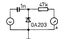
Obr. 215. v_f sonda s paralelním jednocestným usměrňovačem
