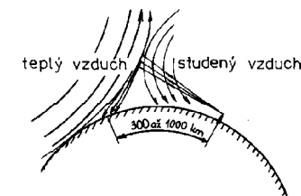
Obr. 244. Příklad šíření odrazem od rozhraní vzdušných front v letním období
