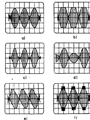
Obr. 175. Průběh signálu při dvoutónové zkoušce: a) nezkraslený SSB signál, b) přebuzený SSB signál, c) špatně nastavený pracovní bod, d) pronikání nosné, e) pronikání nežádoucího postranního pásma, f) zakmitávání
