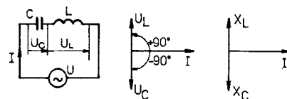
Obr. 33. Sériové zapojení kombinace LC v obvodu střídavého proudu, vektorový součet napětí a reaktancí
