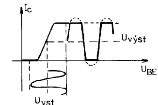
Obr. 114. Princip omezení na charakteristice tranzistoru
