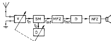
Obr. 146. Blokové schéma přijímače s přímým zesílením
