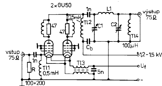
Obr. 173. Koncový vř zesilovač pro KV pásma s elektronkami v zapojení se společnou mřížkou
