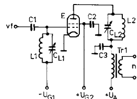
Obr. 96. Amplitudově modulovaný vf zesilovač s elektronkou (anodová modulační)
