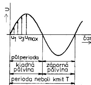
Obr. 9. Sinusový průběh střídavého napětí U a základní pojmy
