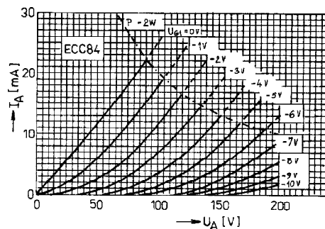
Obr. 57. Příklad charakteristik elektronky z katalogu výrobce
