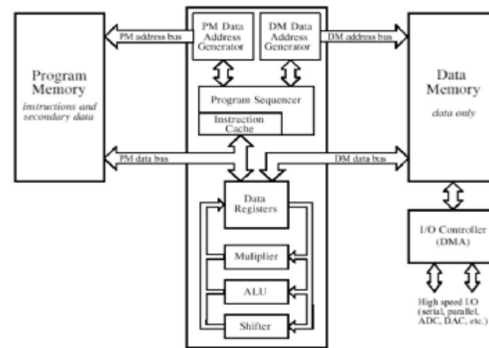
Obr. 153. Blokové schéma DSP
