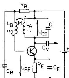
Obr. 91. Zpětnovazební oscilátor s transformátorovou vazbou
