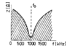
Obr. 118. Kmitočtová závislost impedance sériového LC obvodu
