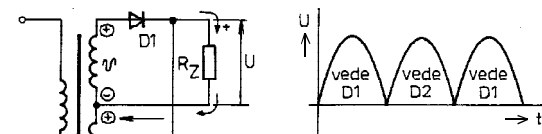
Obr. 46. Dvoucestný usměrňovač s dvojím sekundárním vinutím transformátoru a tvar usměrněného napětí na R_z
