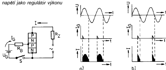
Obr. 71. Tyristor spínající střídavé napětí jako regulátor výkonu
