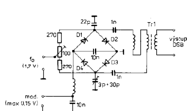
Obr. 97. Balanční modulátor pro amplitudovou modulaci s potlačenou nosnou
