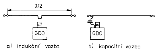
Obr. 223. Měření rezonančního kmitočtu antény pomocí GDO
